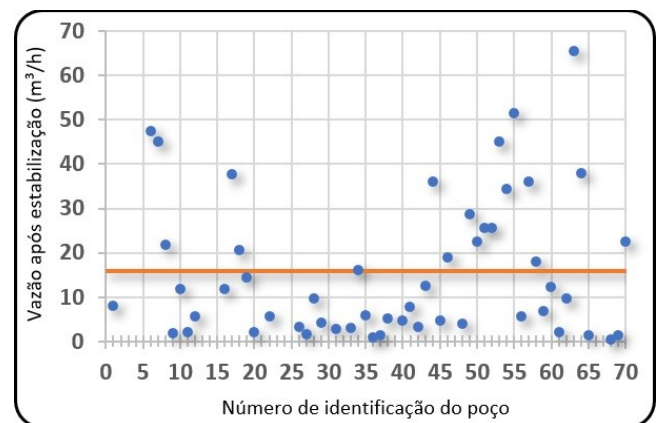
Figure 3 – Vazão após estabilização (pontos na cor azul) e o valor da média 15,77 m³/h (linha na cor laranja).
