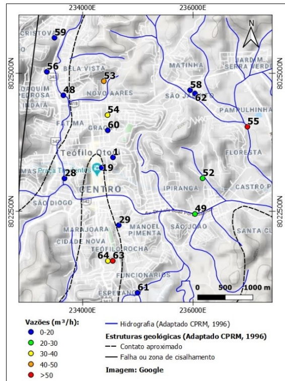
Figura 6 – Área urbana de Teófilo Otoni com a rede hidrográfica (linhas na cor azul). A faixa de vazão para cada poço é indicada pela cor do círculo.
