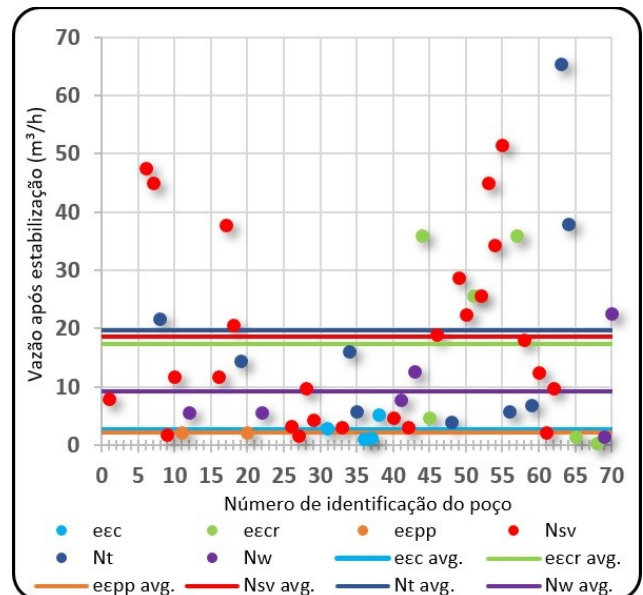
Figura 5 – Vazão após estabilização (pontos) e as média em cada formação geológica (linhas).
