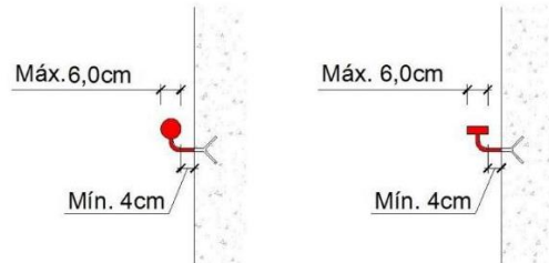
Figura 3 – Pormenores de corrimãos (IT 08 CBMMG, 2020).
