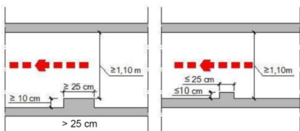
Figura 1 – Medida da largura em corredores e passagens (IT 08 CBMMG, 2020).
