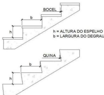
Figura 2 – Altura e largura dos degraus (escada com ou sem bocel) (IT 08 CBMMG, 2020).
